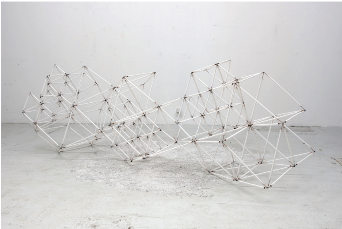
Géométrie cristalline , 2018
